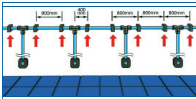
Fase 1: systeem zonder druk
