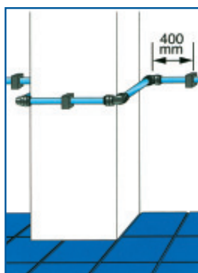
Zuil kleiner dan 1 m
