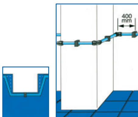
Zuil groter dan 1 m
